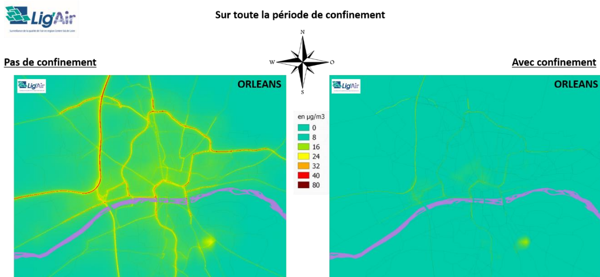
Figure 8 : Evolution spatiale des concentrations moyennes en NO 2 sur Orléans Métropole (concentrations moyennes simulées sur la période du 18 mars au 10 mai 2020 suivant les deux situations (« sans confinement » et « avec confinement »)
