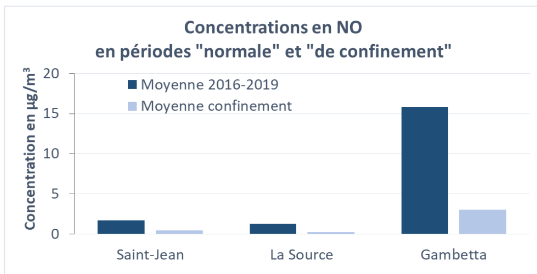
Figure 4 : comparaison des concentrations moyennes en monoxyde d'azote (NO) sur l'agglomération orléanaise durant le confinement et en période « normale »
