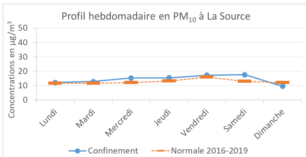
Figure 6 : Profils hebdomadaires en en particules en suspension (PM 10 ) sur le site urbain de fond de La Source à Orléans
