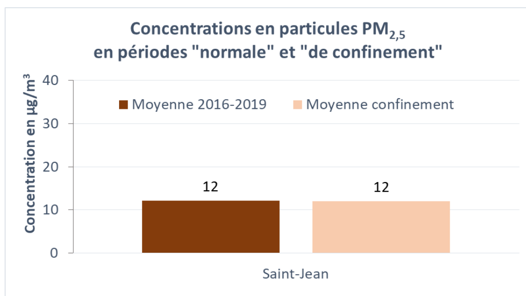
Figure 7 : comparaison des concentrations moyennes en particules en suspension (PM 2,5 ) sur l'agglomération orléanaise durant le confinement et en période « normale »
