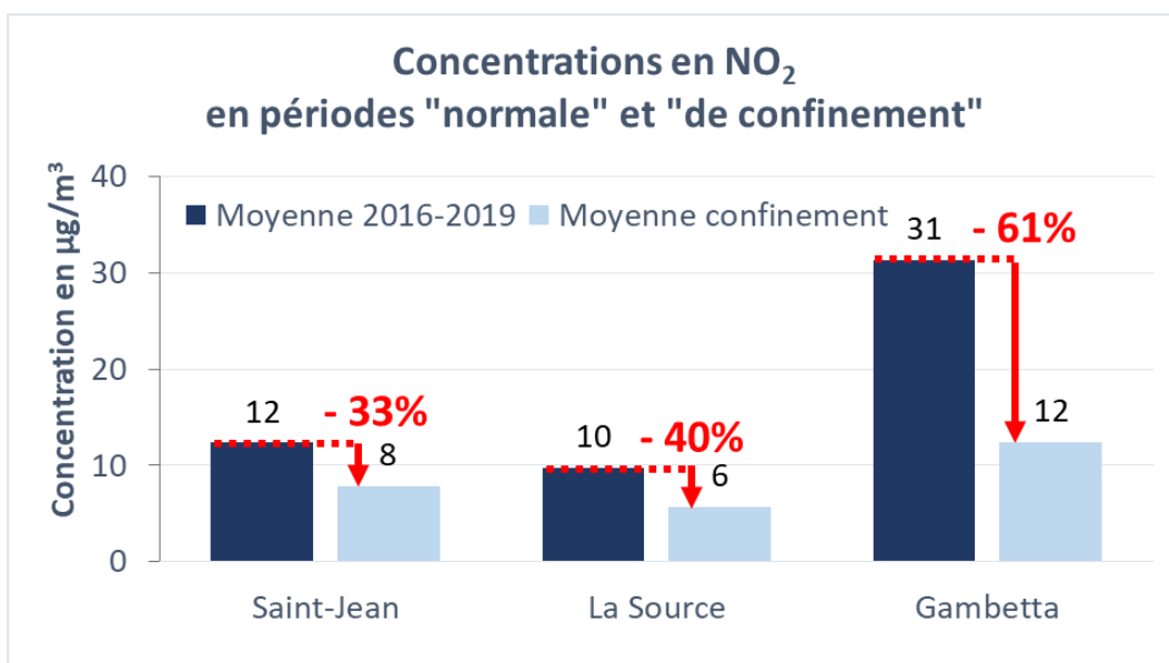
Figure 1 : comparaison des concentrations moyennes en dioxyde d'azote (NO 2 ) sur l'agglomération orléanaise durant le confinement et en période « normale »
