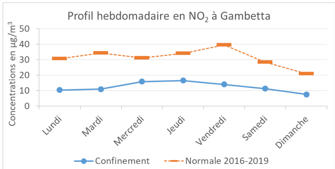
Figure 2 : Profils hebdomadaires en dioxyde d'azote (NO 2 ) sur le site trafic de Gambetta à Orléans
