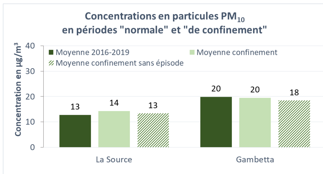
Figure 5 : comparaison des concentrations moyennes en particules en suspension (PM 10 ) sur l'agglomération orléanaise durant le confinement et en période « normale »
