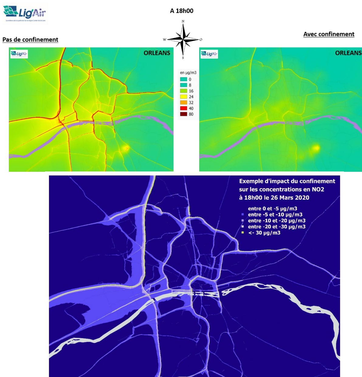
Figure 9 : Concentrations horaires en NO 2 obtenues à 18h00 le Jeudi 26 mars (a) sans confinement et (b) pendant le confinement et (c) carte de différence, sur le territoire d'Orléans Métropole
